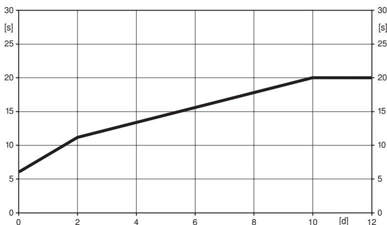
Tempo tipico di pre-carica
